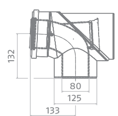
Tronchetto ispezione
