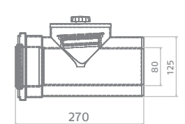
Tronchetto ispezione
