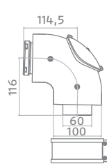
Curva 90° ispezionabile
