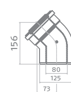
Curva 45°
